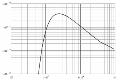
Рис. 1.4. Додаткова об'ємна активність \alpha -випромінюючих радіонуклідів в повітрі (Бк/м 3 ) при фрагментації ферми залежно від відстані (м) від точки викиду
